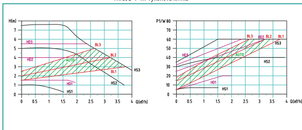
• TRICOE-7.5 III výkonová křivka
